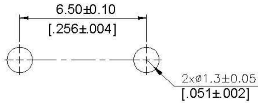
P.C.B. LAYOUT
